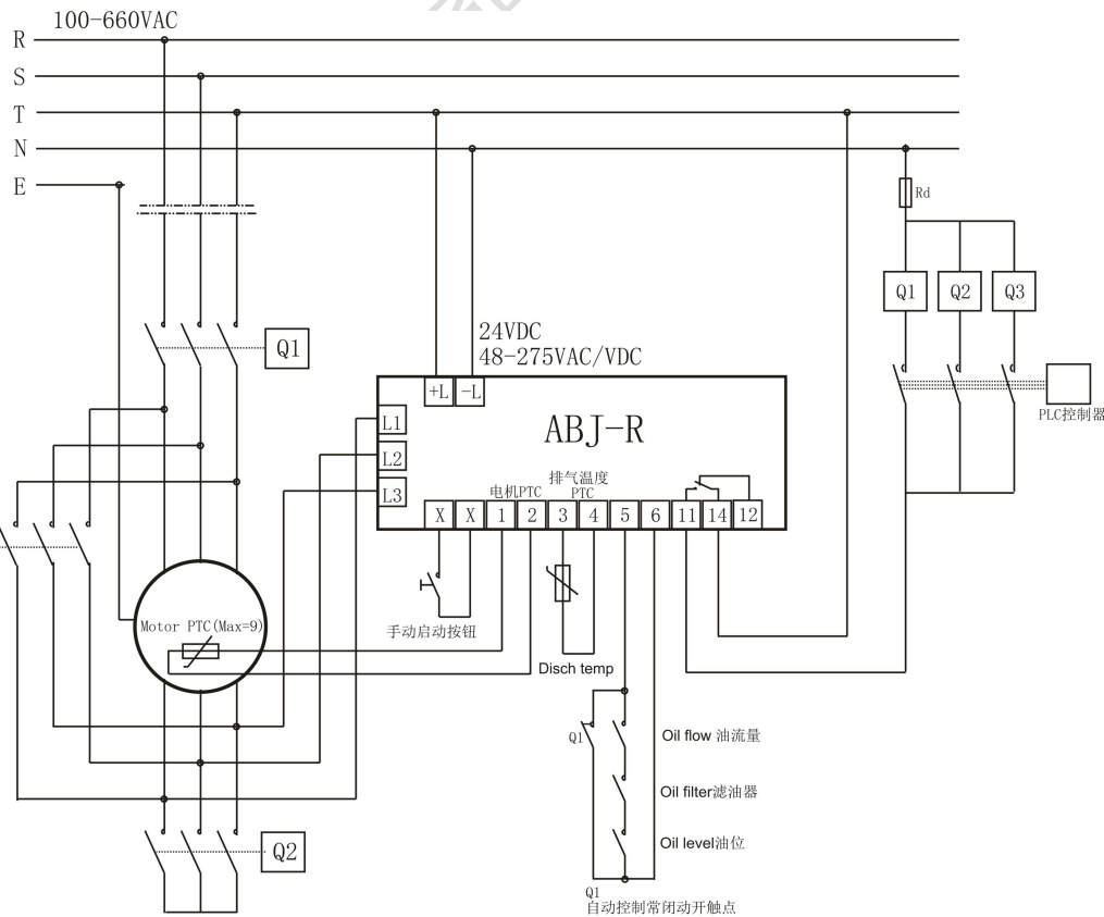
推荐电路 2：Y~△起动电路
